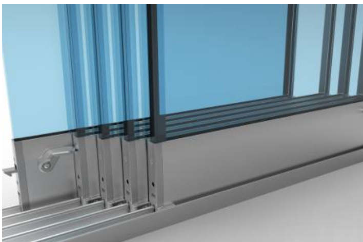
Guía inferior de superficie
