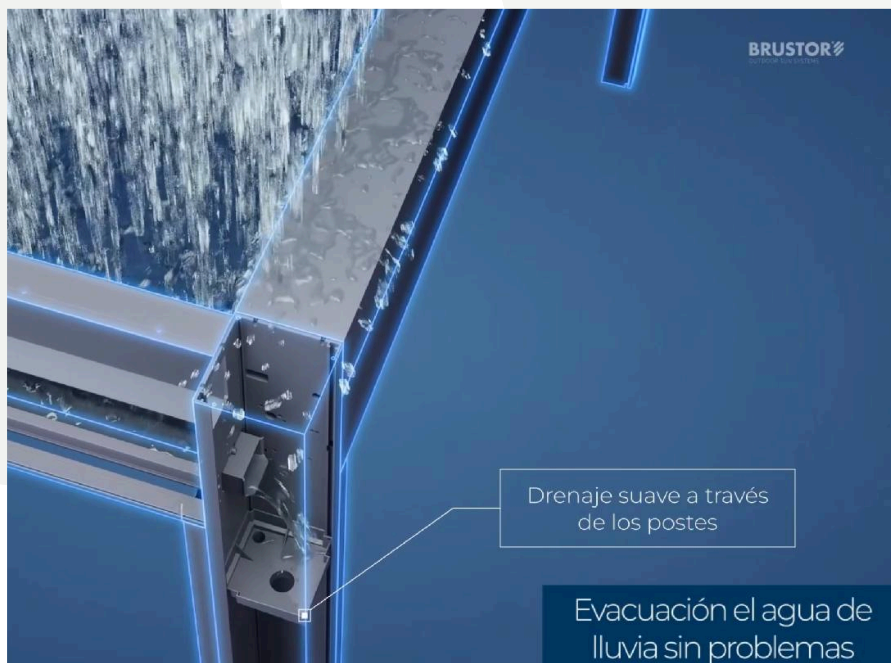
Canalón perimetral con evacuación por el interior de los pilares
