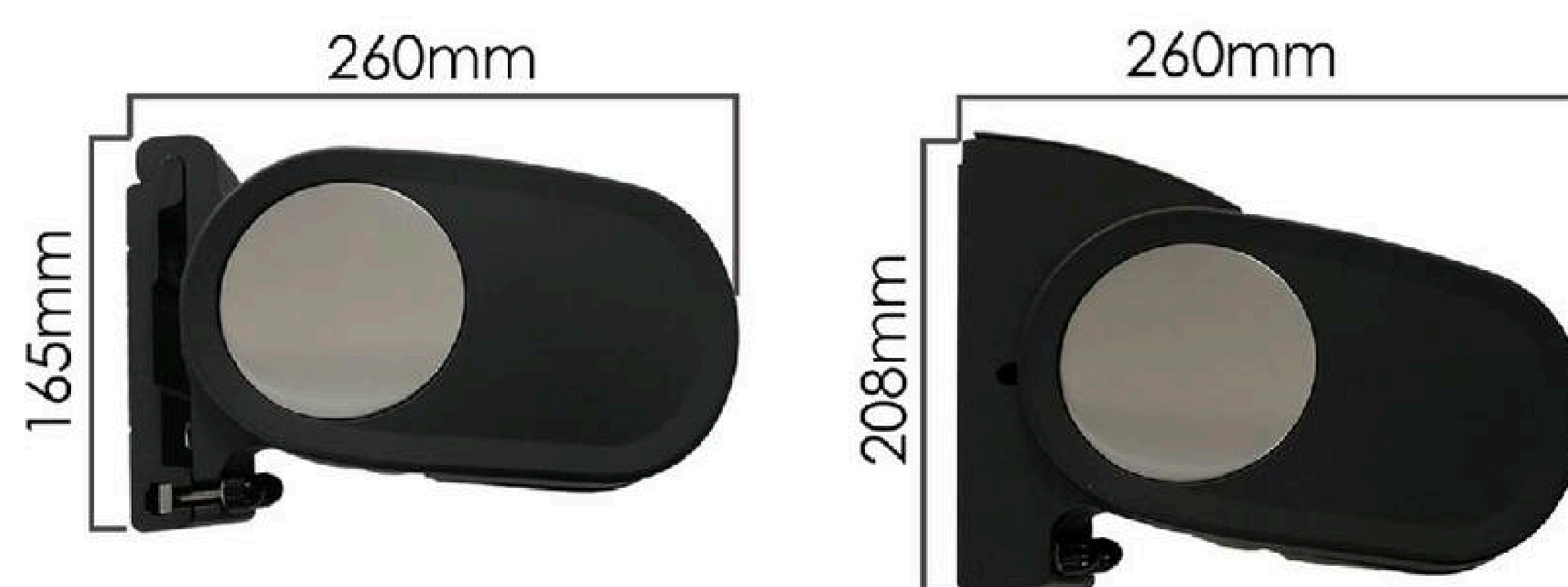
Dimensiones del cofre sin/con tejadillo opcional
